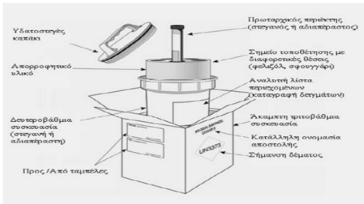
Εικόνα 1. Τριπλή συσκευασία για τη μεταφορά μολυσματικής ουσίας κατηγορίας B.
